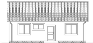
POHLED ZADNÍ
