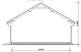
POHLED BOČNÍ - PRAVÝ
