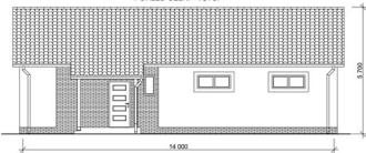
POHLED ČELNÍ - VSTUP
