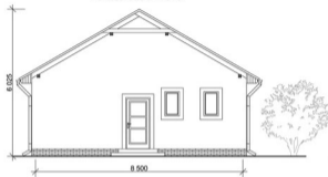
POHLED ČELNÍ - VSTUP
