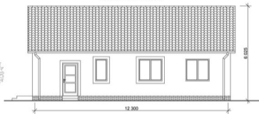
POHLED BOČNÍ - PRAVÝ
